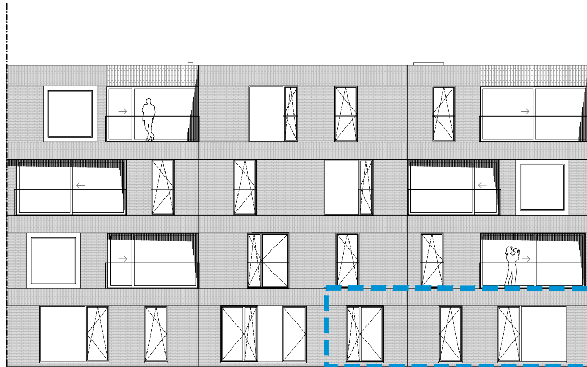
VOORGEVEL
